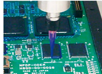
ディスペンサーによる部分塗布（一例）
