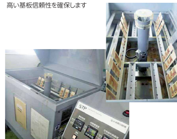
試験条件：JIS Z 2371（ISO9227準拠）500時間
